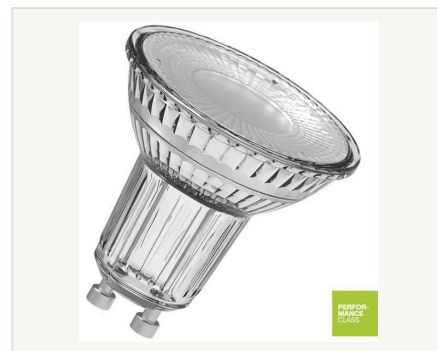
Светодиодная лампа OSRAM GU10 2,4W 2700K 220V 230Lm 36°
