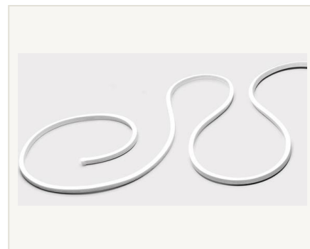
Светодиодная подсветка Neon flex strip 7,2W/m 3000K
